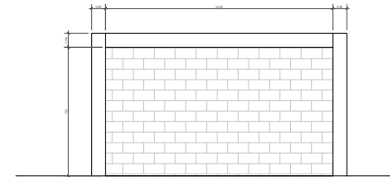
DETALLE DE MURO PERIMETRAL
